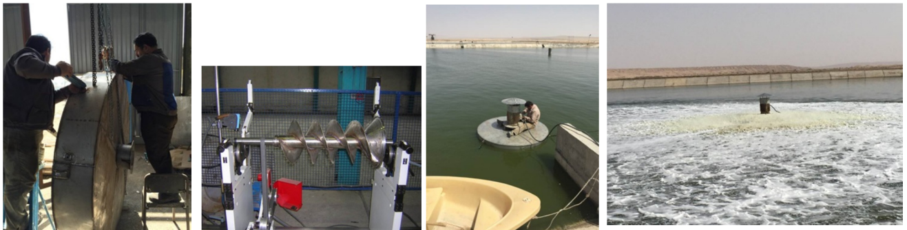
ساخت دستگاه هواده دور تند تصفیه خانه فاضلاب شهر سمنان ( استان سمنان)
